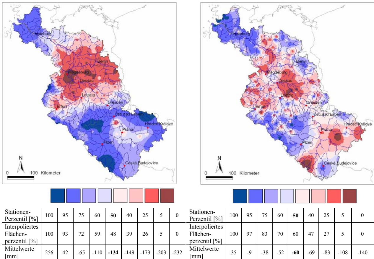
a. KWB Mittelwerte Sommer
