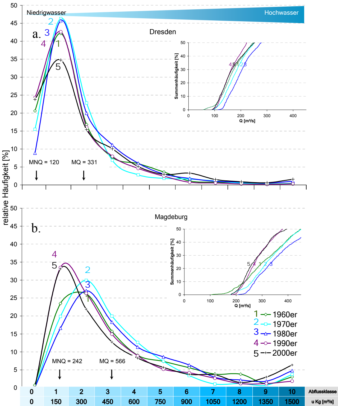
Abb. 5a,b,c,d: Mittelfristige Veränderungen in der Häufigkeit von Abflussklassen und der Summenhäufigkeit von Abflüssen analog zu Abb. 4 an den Pegeln Dresden (a), Magdeburg (b), Barby (c) und im Mittel (d) über 8 Elbpegel (vgl. Tabellen 2 und 3)
