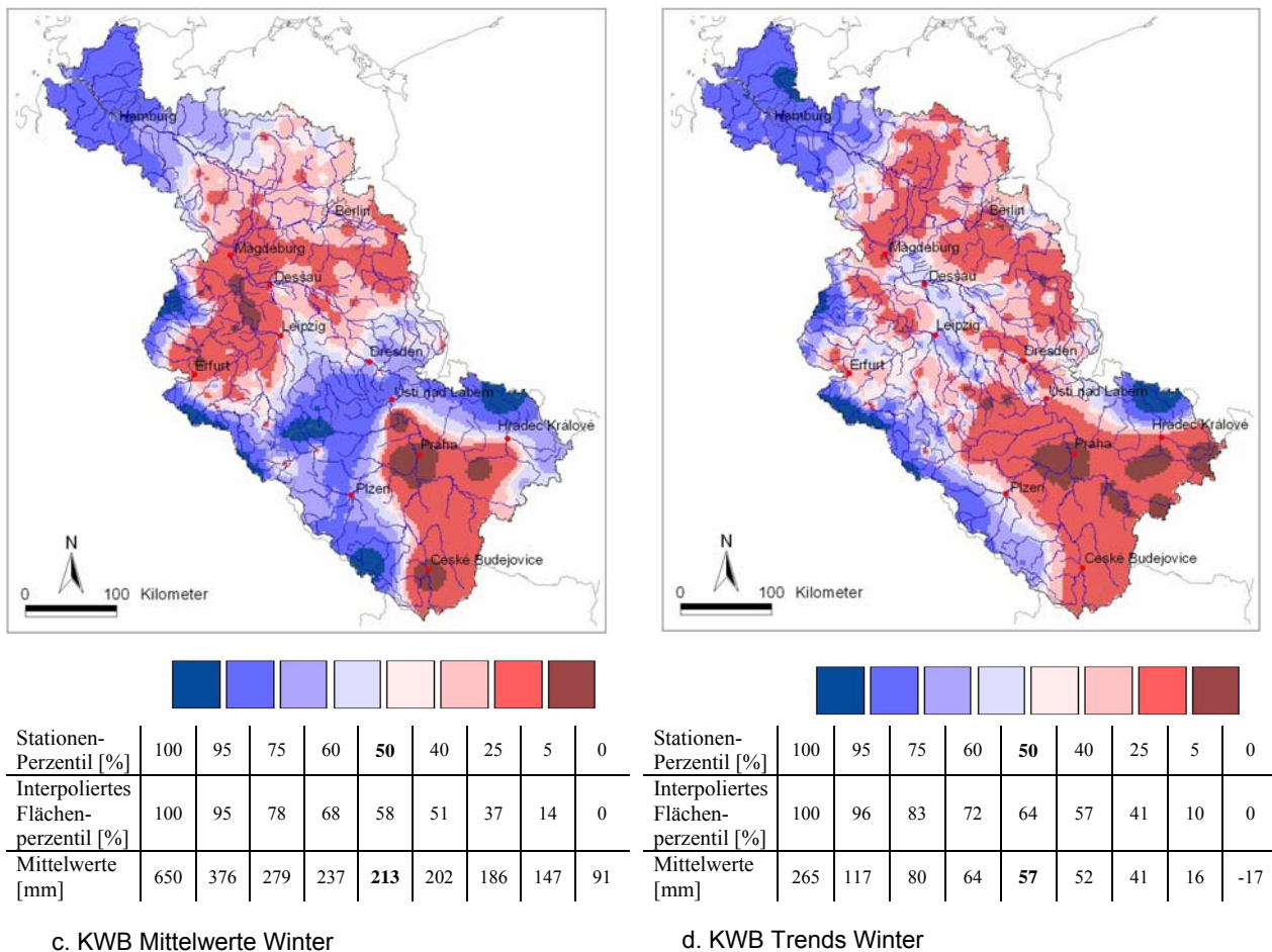
Abb. 17c, d: Mittelwerte (c) und mittlere Trends (d) der klimatischen Wasserbilanz im Zeitraum 1951-2000 für den hydrologischen Winter analog zu Abb. 17a, b. Die Zentralwerte (50% Perzentil) der Stationsmittel und der Stationentrends für den Winter lauten 213 mm und 57 mm. Die Zentralwerte der interpolierten Halbkilometer Rasterwerte liegen bei ca. 202 und 50 mm.
