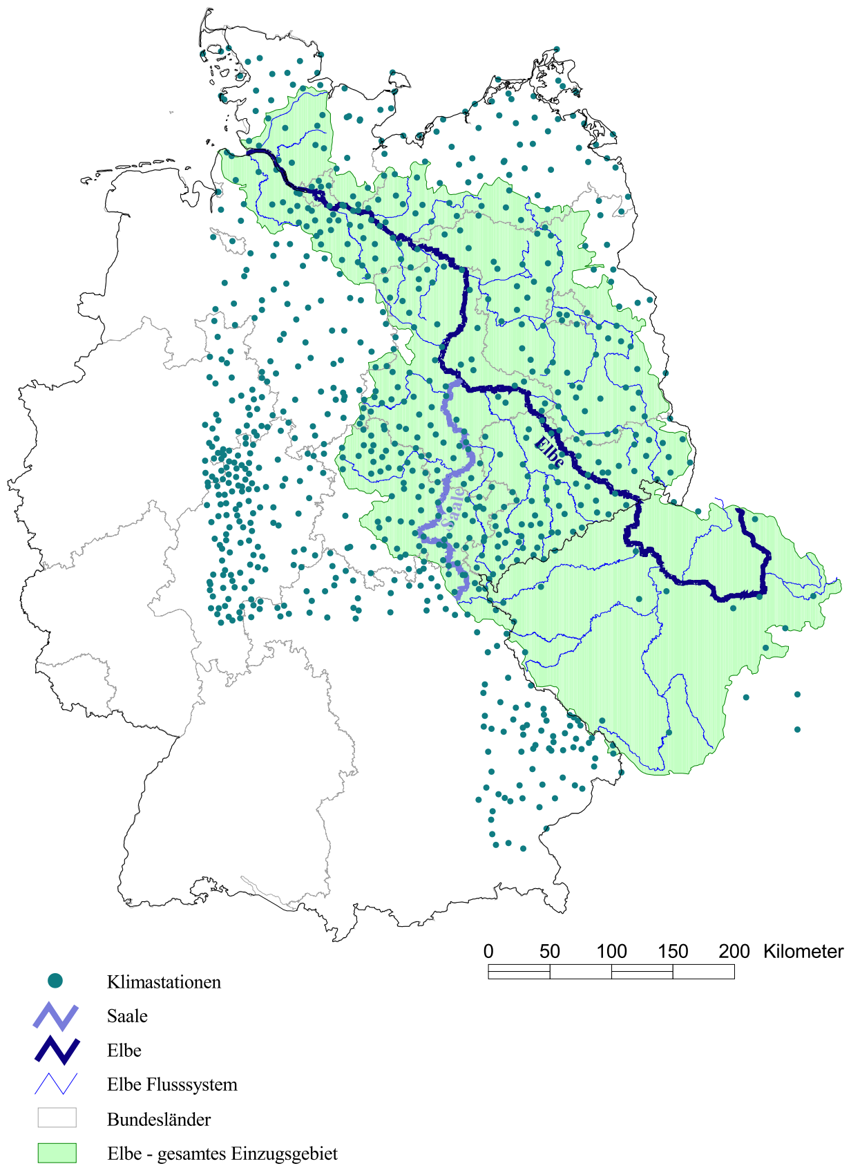
Abb. 3: Klimastationen und Niederschlagsbeobachtungspunkte auf deutschem und tschechischem Gebiet für die Analysen zur klimatischen Wasserbilanz
